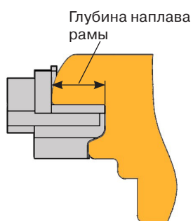
Торцевая накладка с углом 90^\circ
