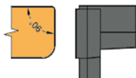
Торцевая накладка с углом 90^\circ
