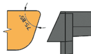
Торцевая накладка с углом 75-85^\circ
