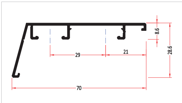
Профиль на створке 70/28, ALUSTART PLUS, (6 м)
