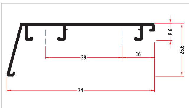
Профиль на створке 74/26, ALUSTART PLUS, (6 м)
