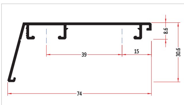
Профиль на створке 74/30, ALUSTART PLUS, (6 м)
