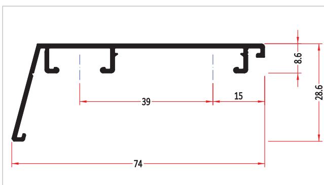
Профиль на створке 74/28, ALUSTART PLUS, (6 м)
