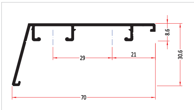
Профиль на створке 70/30, ALUSTART PLUS, (6 м)
