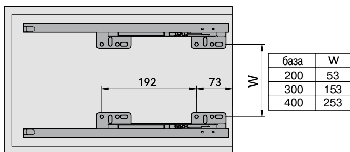
Установка направляющих
