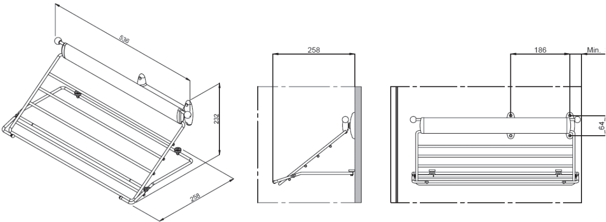
Габаритные и установочные размеры брючницы VIB0229
