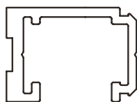
35 Верхняя направляющая на раме
