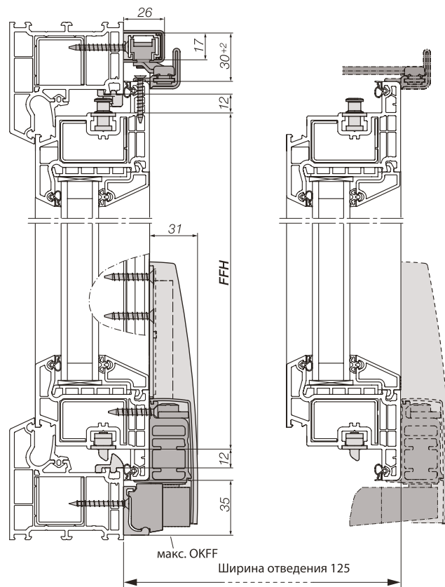
Разрез по вертикали, Internika HKS 160 S пластик
