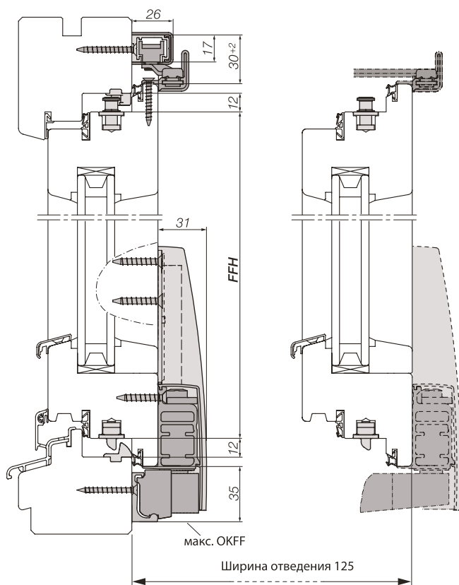
Разрез по вертикали, Internika HKS 160 S дерево
