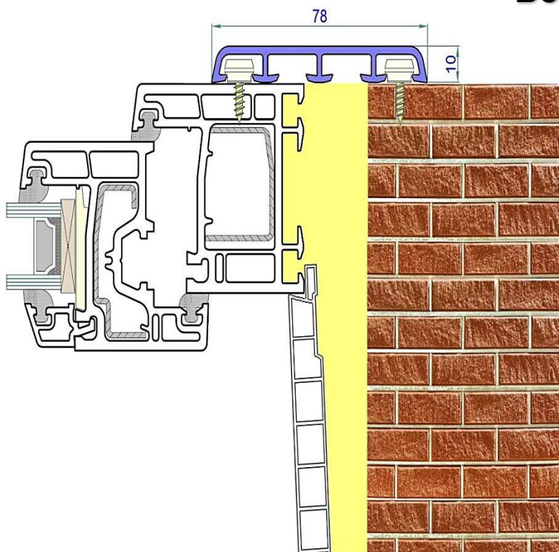
Заподлицо
