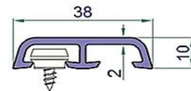
Нащельник 38 мм
