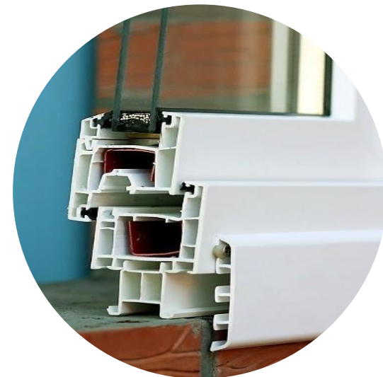
Боковое примыкание
