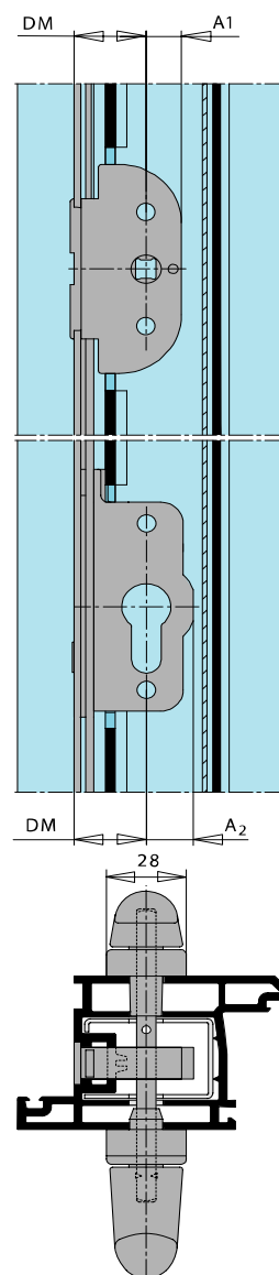
Пластиковый профиль
