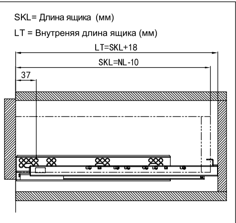
Размер ящика (мм)
