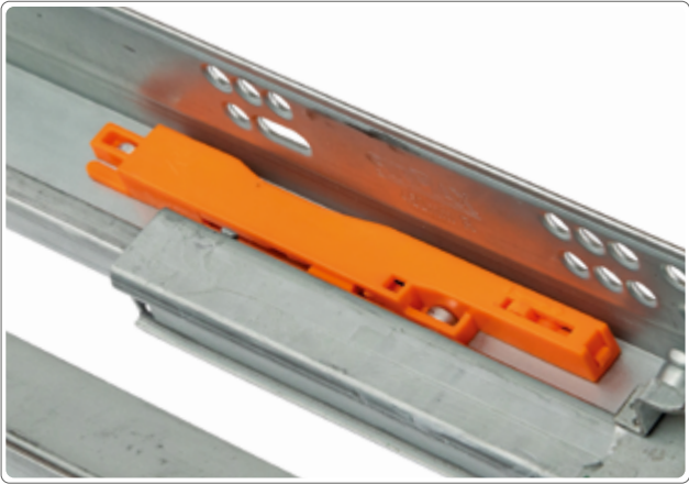
Комплект направляющих скрытого монтажа Firmax 3D Control с механизмом PUSH-TO-OPEN
