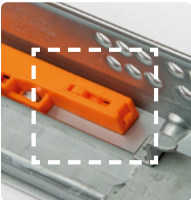
Регулировка усилия открывания ящика
