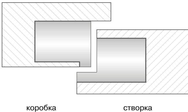
С наружным фальцем
