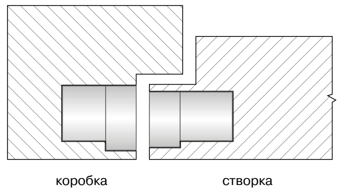
Нефальцованное заподлицо / с внутренним фальцем
