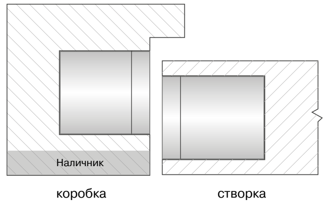
Нефальцованное заподлицо с наличником
