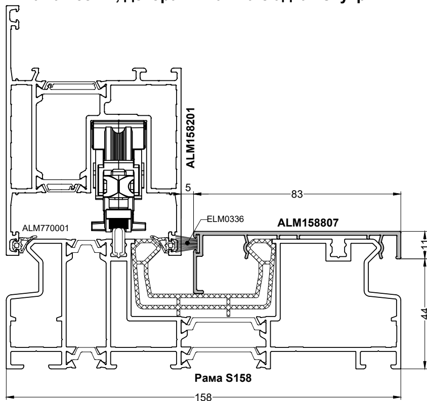
Рама 158мм, декоративная накладка изнутри
