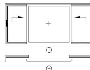
Схема K/1
