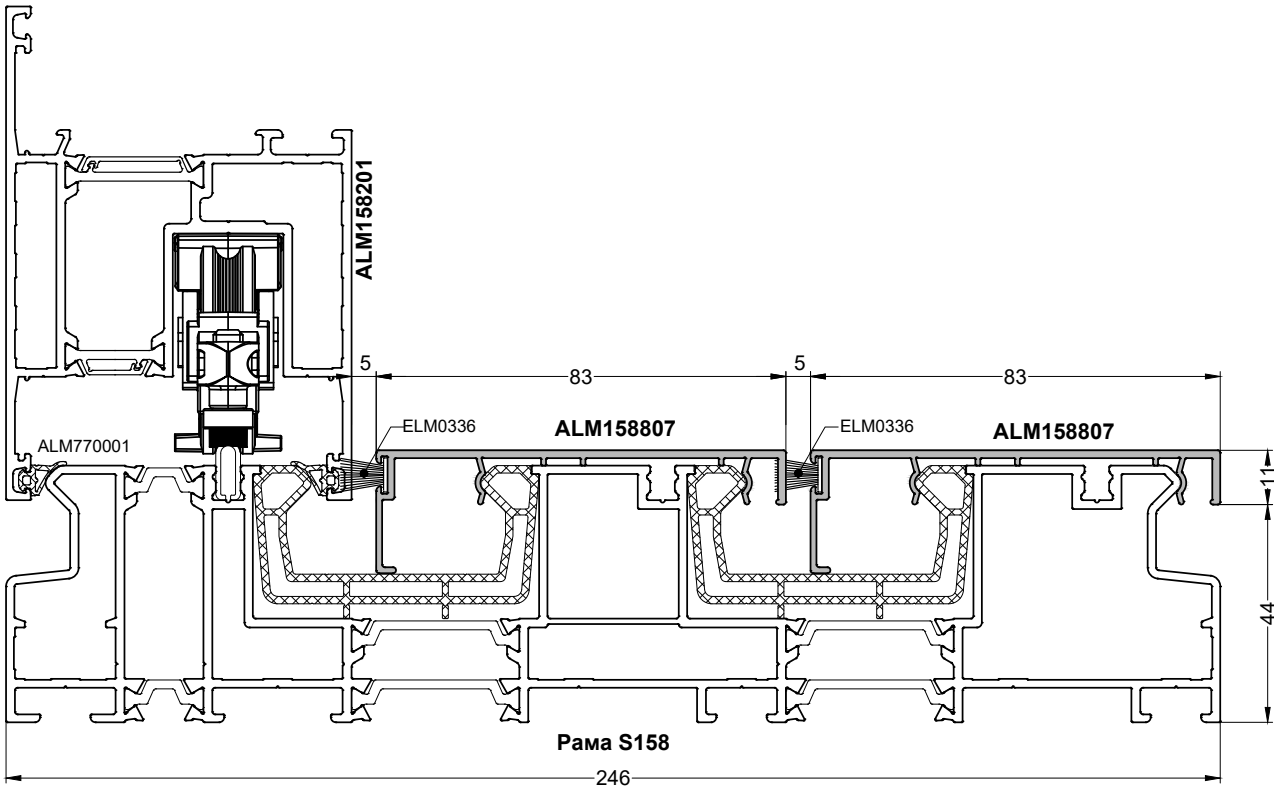
Рама 246мм, декоративная накладка изнутри
