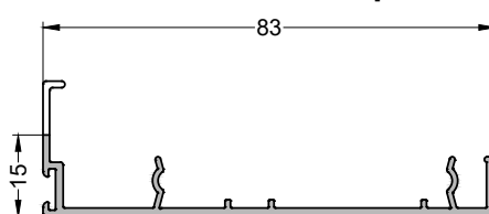
Соединение ALM158807 со створкой
