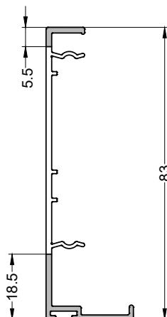
Соединение ALM158807 с рамой
