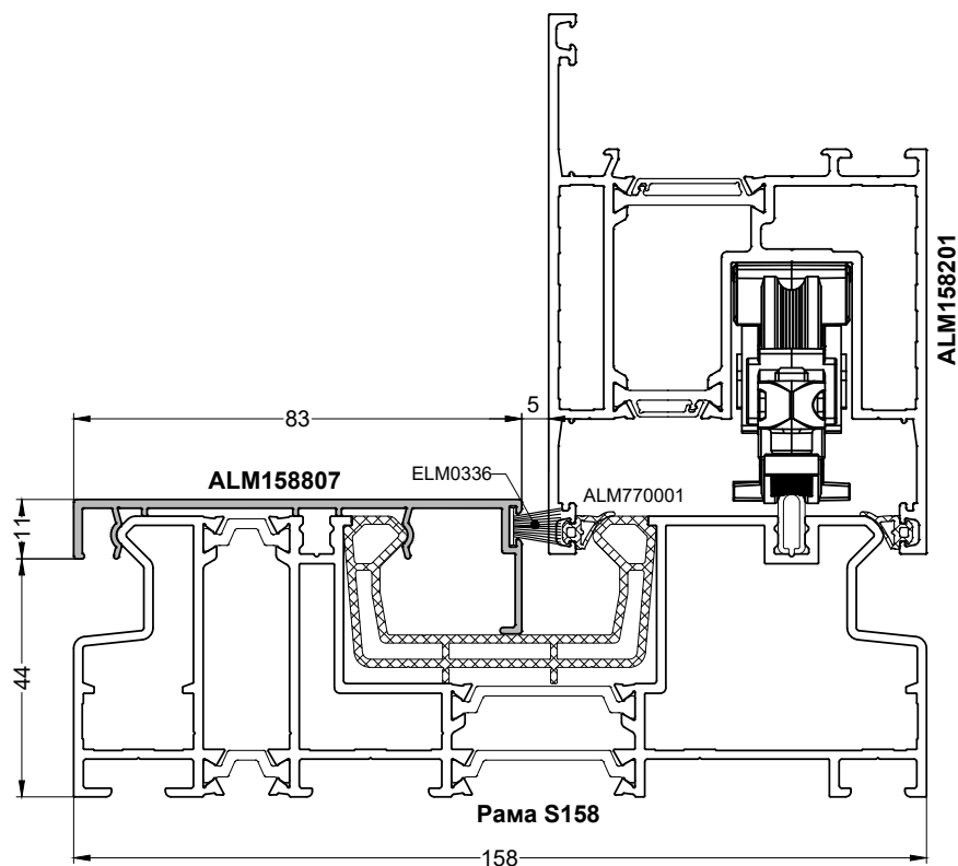
Рама 158мм, декоративная накладка изнутри
