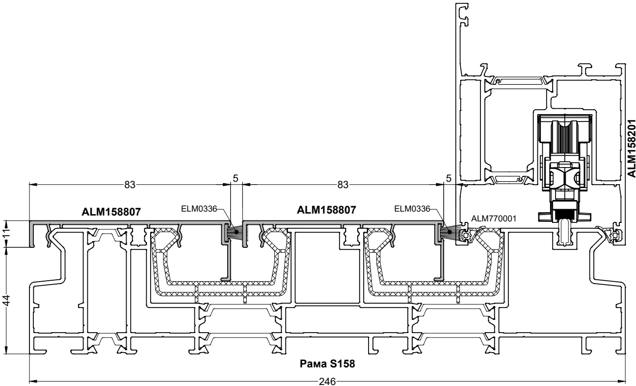
Рама 246мм, декоративная накладка изнутри
