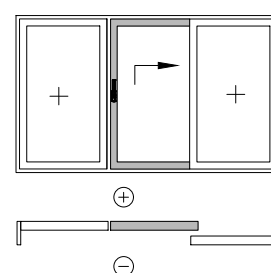
Схема C/1
