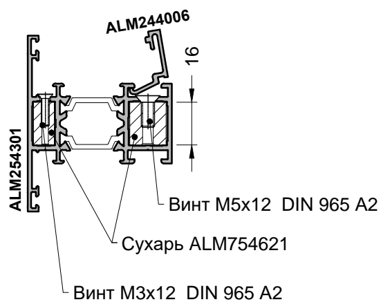
Установка штапика ALM244006 Момент установки в паз
