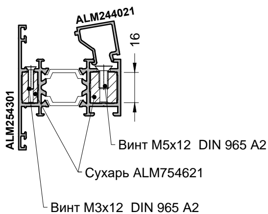
Установка штапика ALM244021 Момент установки в паз
