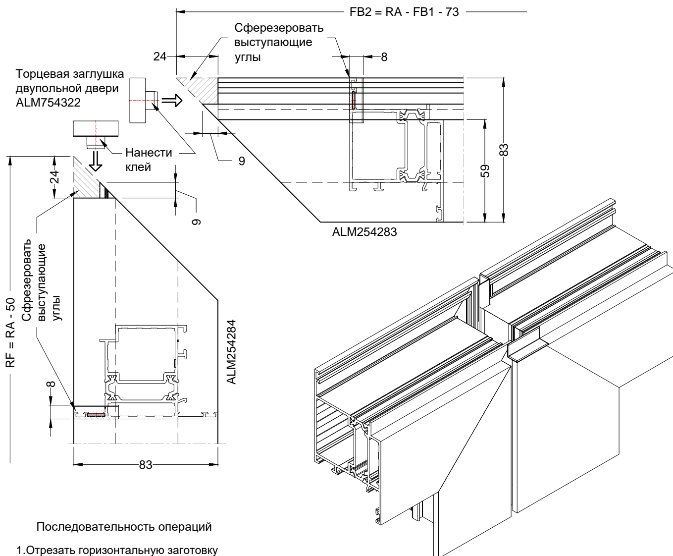
Двупольная дверь с внутренним открыванием
