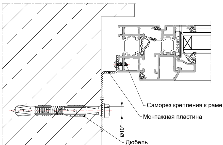
Установка оконной рамы с помощью монтажной пластины
