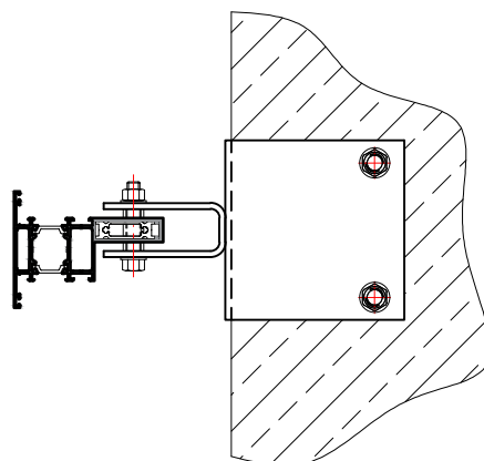
Вид сверху
