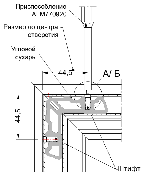
Схема установки штифтов
