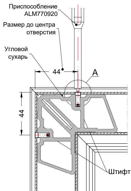
Схема установки штифтов
