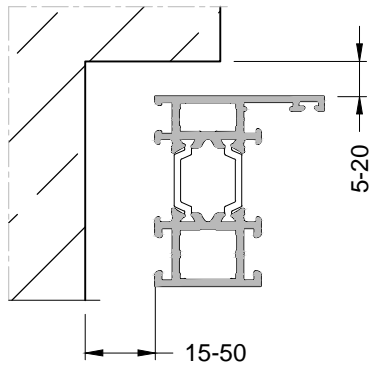
Установка в проем с четвертью
