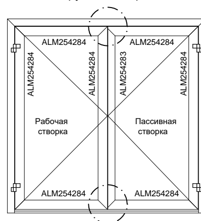
Двупольная дверь с наружным открыванием
