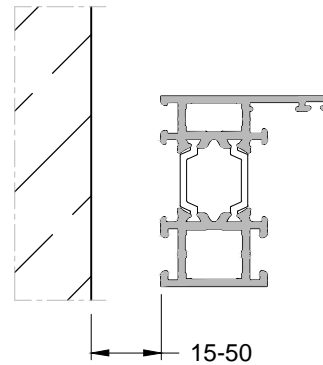
Установка в проем без четверти
