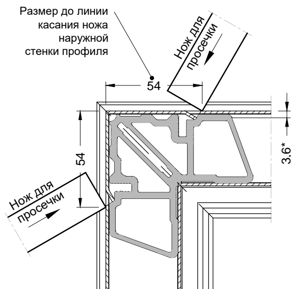
Схема опрессовки угла
